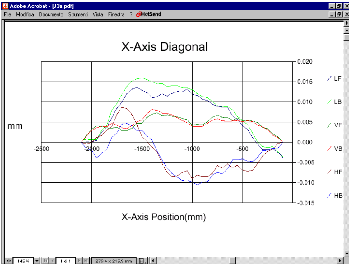
Fig 10 (sopra) errori sull'asse X; le curve superiori sono l'errore di posizionamento lineare, le curve centrali l'errore di rettilineità verso Y e le curve inferiori sono l'errore verso Z Fig 11(sotto) errori sull'asse Y, la curva superiore è l'errore di posizionamento lineare, la curve verde e rossa, l'errore di rettilineità verso X e le curve marrone blu l'errore verso Z
