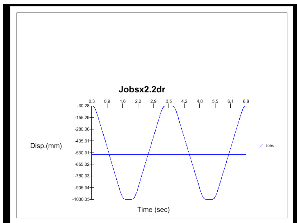
Fig 21 misura di spostamento a gradino con l'uso di una specchio di 3mm di diametro per annullare le vibrazione di eventuali supporti. Spostamento 1m lungo Y feed 50m/min
