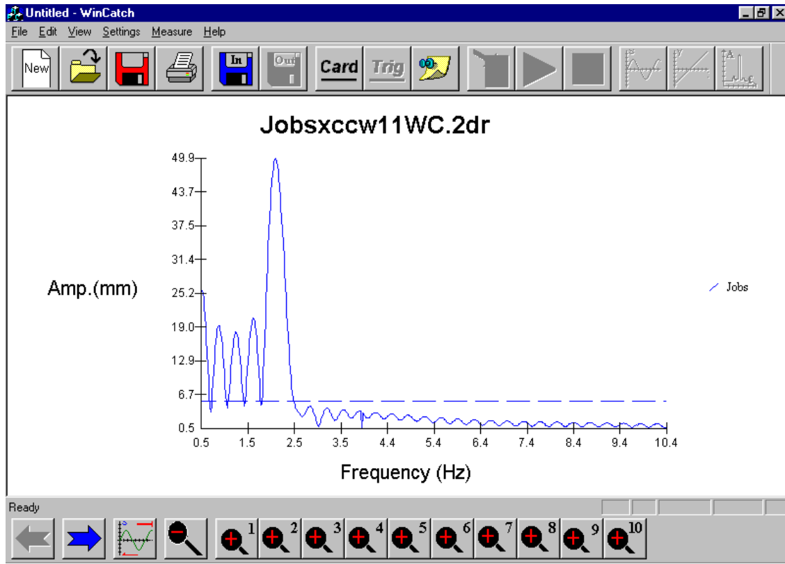
Fig 20 Frequenza dalla misura della laser Ballbar . La presenza di una sola frequenza, quella di rotazione(non si nota la presenza di seconda o della terza armonica) significa distorsione quasi nulla ne distorsioni armoniche del movimento degli assi. Questa raffigurazione nel dominio delle frequenze riassume con buona approssimazione i risultati delle tre figure precedenti.
