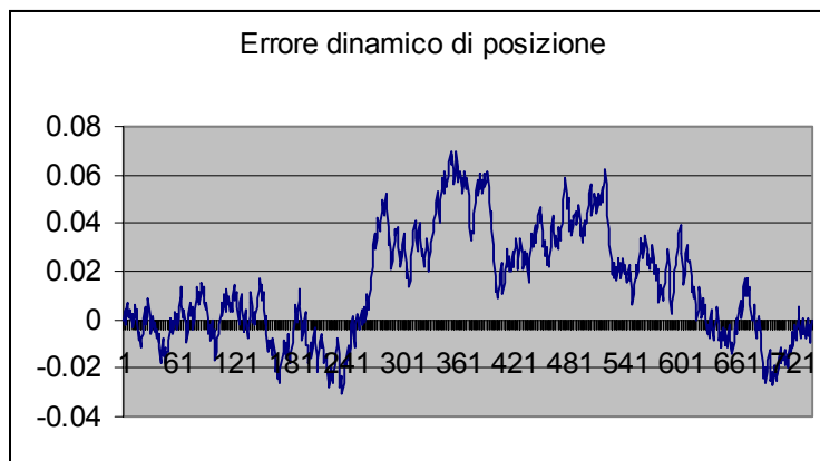
Fig. 27 errore di inseguimento per movimento a velocità uniforme. Scala in mm e milli secondi
