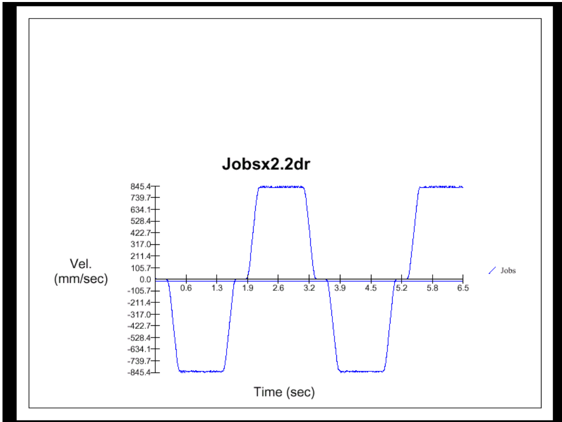
Fig 23 grafico di velocità
