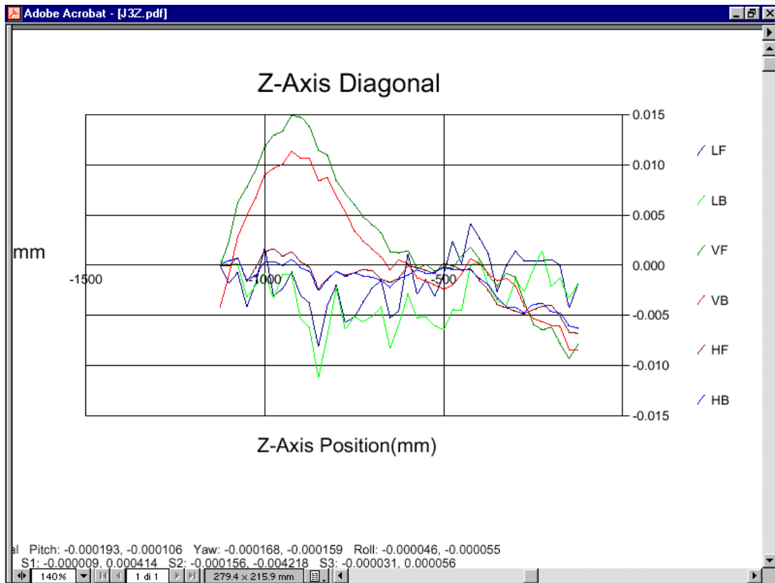
Fig 12 errori relativi all'asse Z LF ed LB sono l'errore lineare, VF e VB sono l'errore di rettilineità in direzione di X e HF ed HB sono l'errore di rettilineità in direzione Y.
