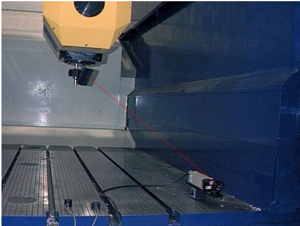
Fig . 7 Misura diagonale per passi con specchio piano sul mandrino e laser sulla tavola.
