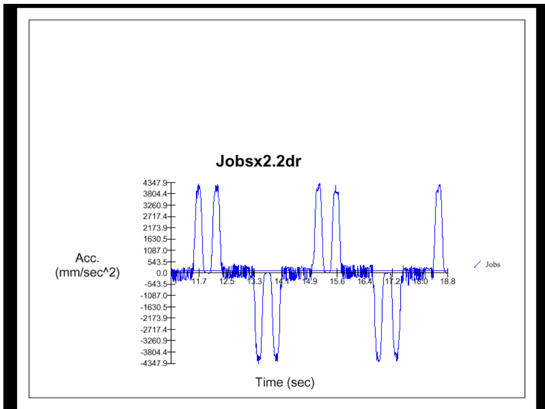
Fig 26 accelerazione durante la fase di spostamento a gradino . Si può notare che i due picchi successivi , rispettivamente di frenata e accelerazione si superano 0,4 g.
