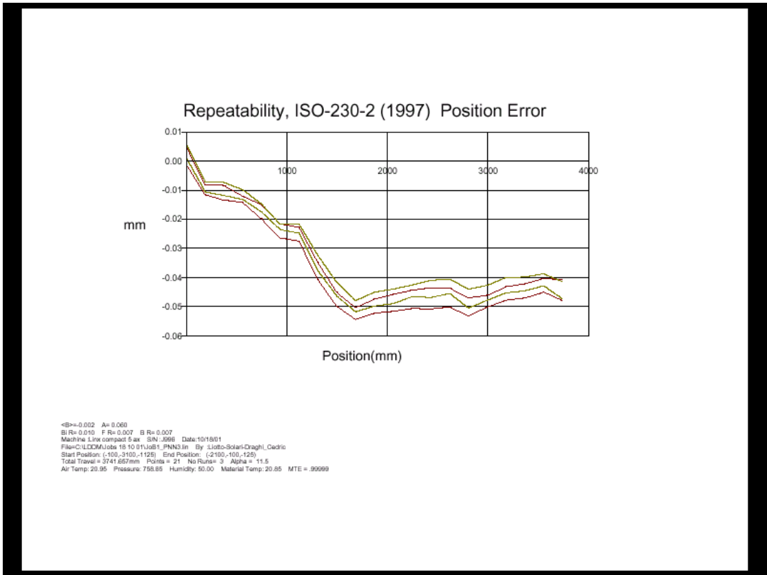
FIG 5 Misura statistica effettuata sulla diagonale PNN effettuata 3 volte in ogni direzione. ed analizzata secondo la ISO230 con deviazione 2 sigma. Fig 6 Errore di inversione lungo tutti punti della diagonale
