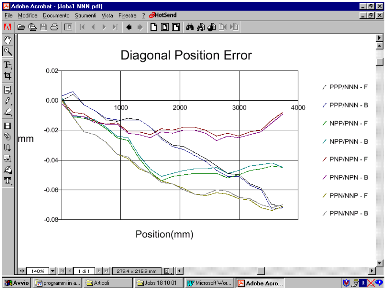
Fig 2 Errore di posizione Volumetrico relativo alle 4 diagonali
