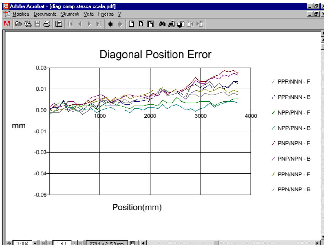
Fig 9 sotto Errore di posizionamento dopo la compensazione (stessa scala) L'errore totale si è ridotto a 30 micron .
