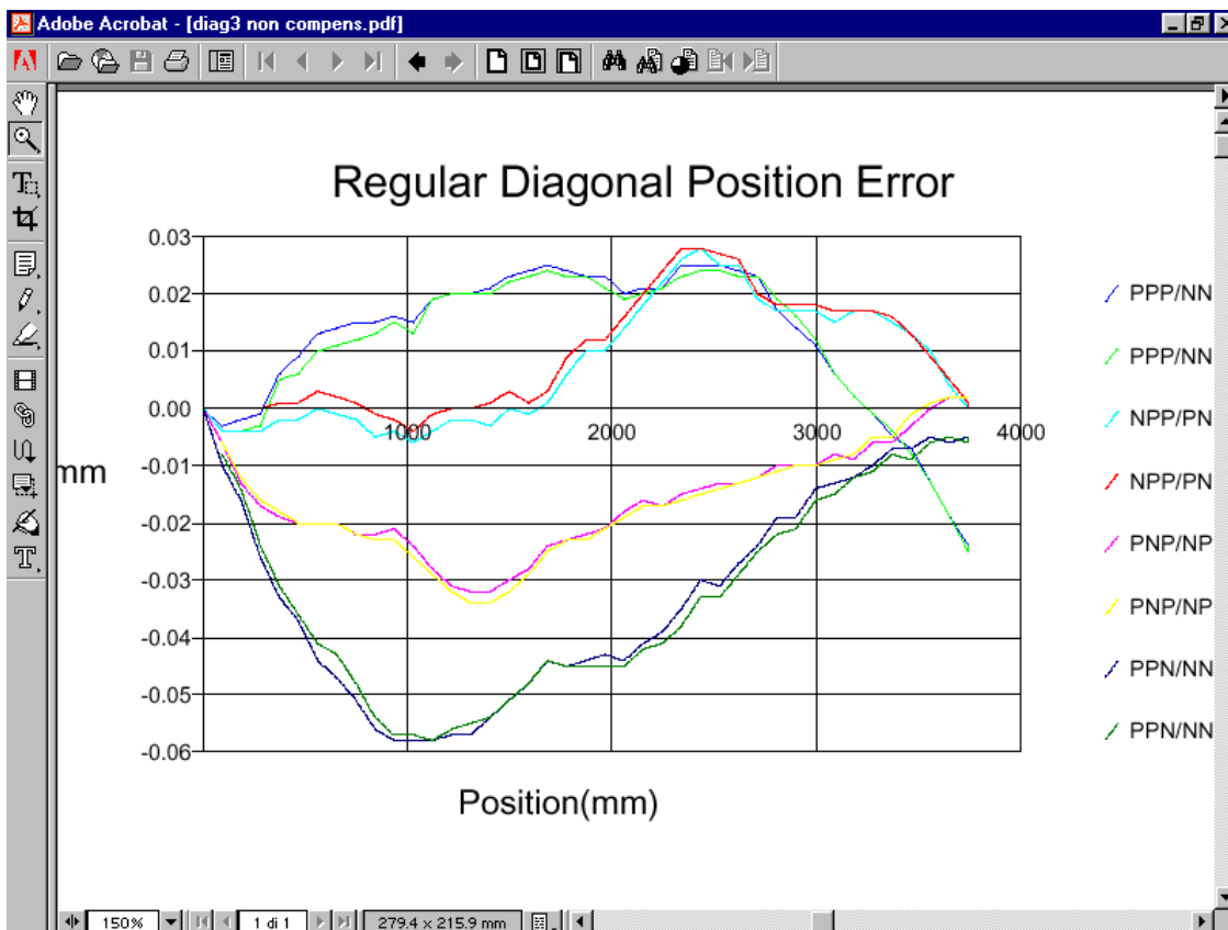
Fig 8 Errore di posizionamento diagonale prima della compensazione . L'errore totale è circa 90 micron.
