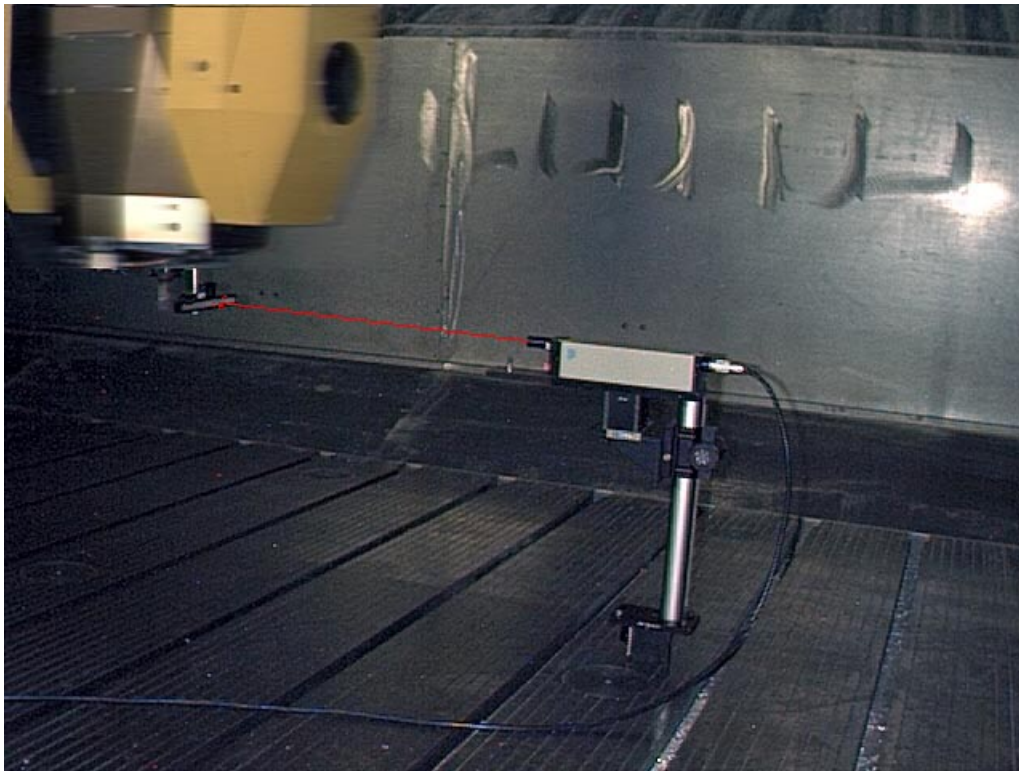
Fig. 15 Misura di interpolazione circolare Laser Ballbar sul piano XY velocità 50000 diam 50mm Fig. 16 Tavola riassuntiva dei risultati della prova del cerchio
