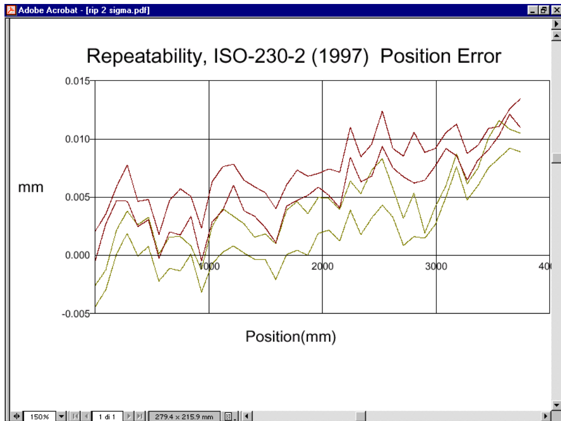
Fig. 14 errore statistico di ripetibilità ottenuto con 3 corse bidirezionali ed elaborazione secondo la ISO-230-2 del 1997 la traccia rossa è la media + e - 2 sigma per la corsa avanti. la traccia gialla +e- 2 sigma per la corsa di ritorno
