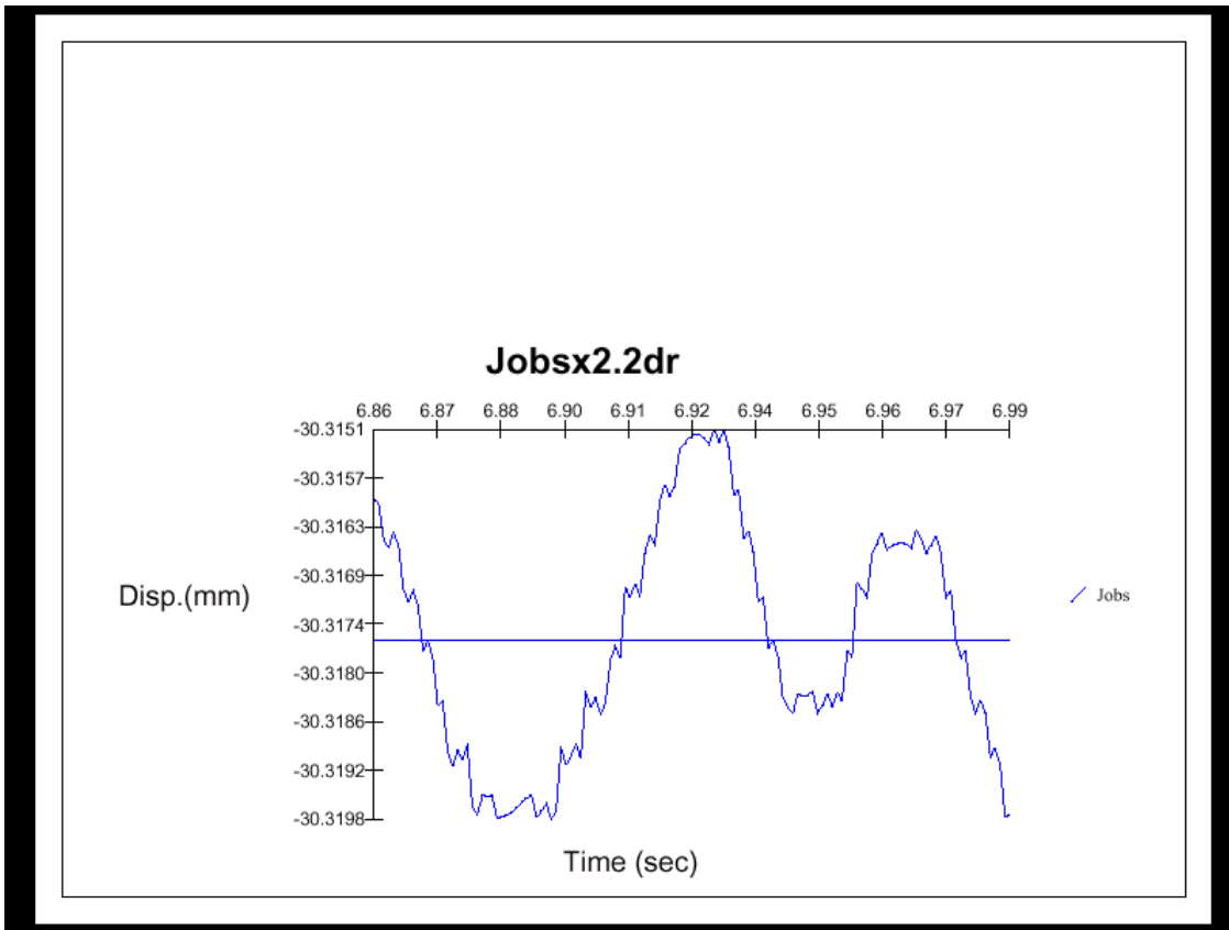
Fig 25 Grafico di posizione durante la fermata zoom X1000
